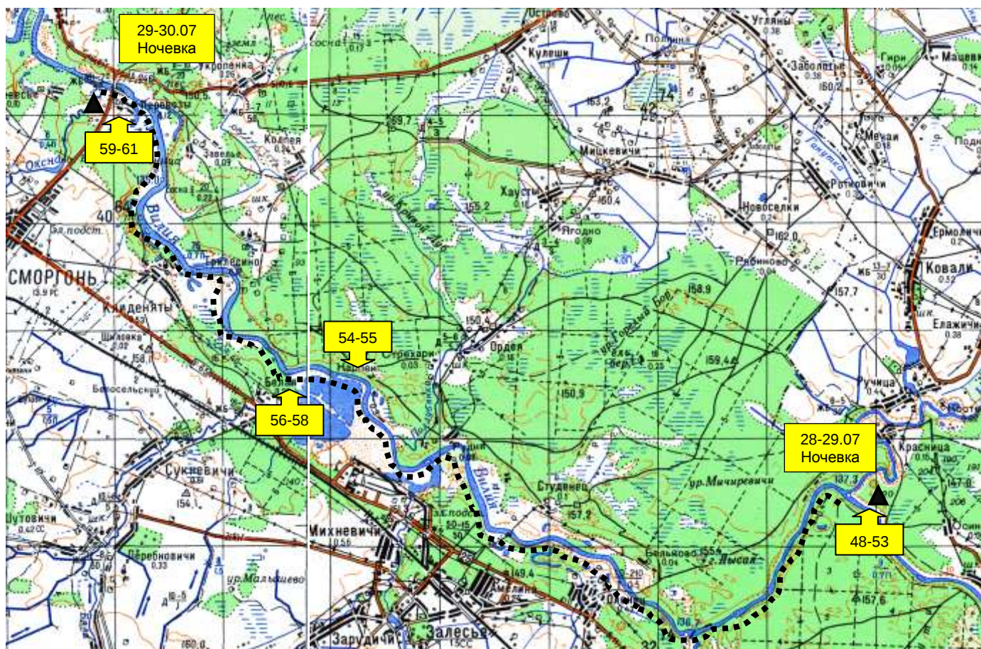
Карта 3 (лоция). М 1:100000 29.07 устье р.Нарочанка – р.Вилия – г.Сморгонь
